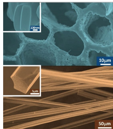
一方凍結法を用いて作製した微細構造のSEM写真: (上) ゼオライトハニカム多孔体、(下) チタニア繊維 ゲル、多孔体、焼結体、粉体等の中での熱及び物質の移動を制御し、特殊な構造や吸着選択性を持つ機能性吸着材の開発を行っています。
