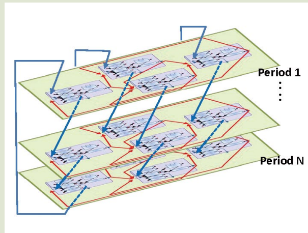
多期間バイオマスサプライチェーンモデル バイオマスの収集から製品化まで、季節性を考慮できるモデルを開発しています。
