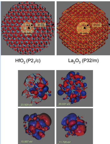
クラスタモデルの電子状態
