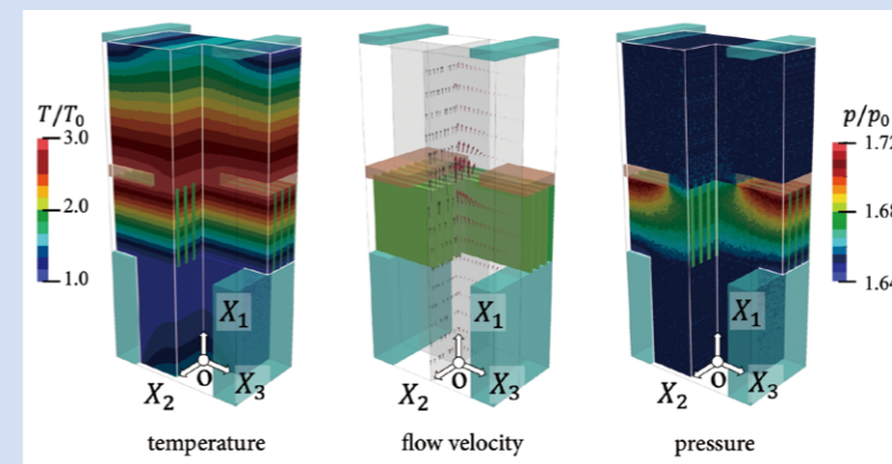
低圧気体やマイクロ流体では、日常の経験に基づく常識に従わない現象も多い。図は、温度差をエネルギー源とする気体の流れや混合気体分離装置への応用。
