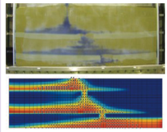
【左図】排水過程における土中間隙流体の形態変化の可視化
