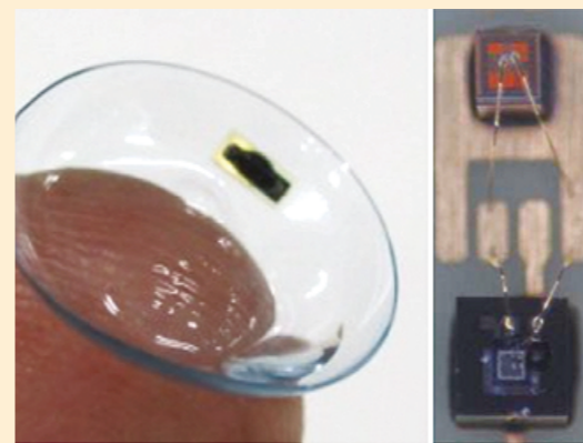
65nm 半導体集積回路チップと糖発電素子を組み合わせた単独動作可能な持続血糖モニタスマートコンタクトレンズ
