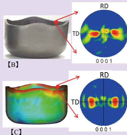
純チタン板の円筒絞り成形の実験と数値シミュレーション
