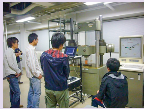
【左写真】岩石の一軸圧縮試験の様子
