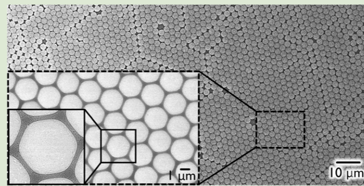
大小 2 種類の微粒子から構成される規則配列単層膜 規則的な粒子配列構造は特異な光学的性質を示すため、簡単に、かつ大面積に粒子膜を製作する方法とそのメカニズムを研究しています。この写真では、小粒子 (直径 45 nm) が大粒子 (直径 2 μm) 同士の隙間に入り込むことで、大粒子が規則的に配列するのを助けています。
