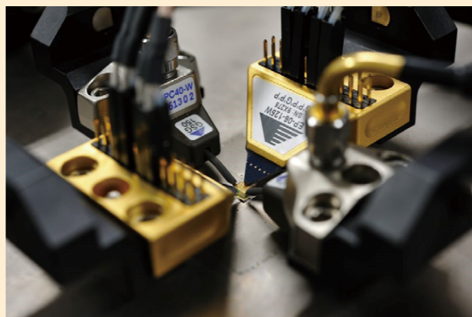
超低電力動作する集積回路の特性評価風景 集積回路デバイスの超低電力動作を目指し、プロセッサをはじめとした様々な集積回路の設計や特性評価を行っています。 【写真】集積回路の特性評価風景
