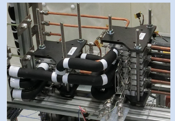
低圧気体やマイクロ流体では、日常の経験に基づく常識に従わない現象も多い。図は、温度差をエネルギー源とする気体の流れや混合気体分離装置への応用。
