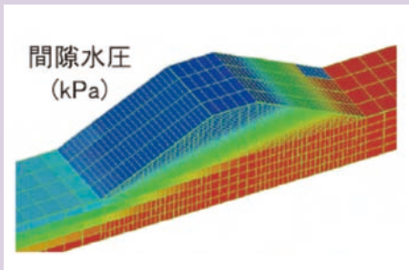
【左図】河川堤防周辺の土構造物の浸透変形解析 地盤の大変形・破壊現象の高精度な予測を実現するために、水と地盤材料の相互作用を伴う力学現象の解明と、そのメカニズムの理解に基づく地盤の変形予測手法に関する研究を実施している。 【右図】土壌・地下水汚染の浄化・リスク評価 土壌や地下水汚染の浄化やリスク評価を実施するために、室内実験や数値解析を通して地盤中での重金属、有機塩素化合物等の挙動評価と対策手法の検討を行っている。
