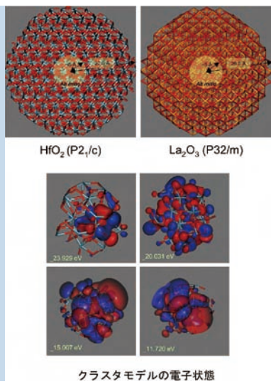
クラスタモデルの電子状態
