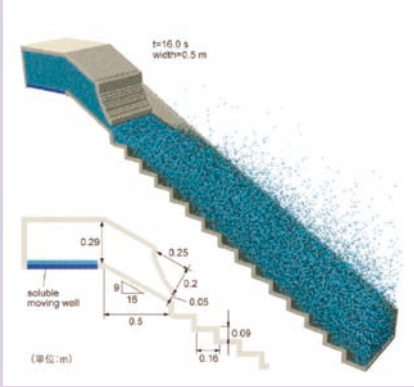
【左図】粒子法による砕波・激流のシミュレーション 水塊の分裂や再合体を伴う複雑な水理現象を再現するために、粒子法による水理シミュレーション手法の開発を行っている。さらに、群集の避難シミュレーション等への粒子法の新たな展開を目指している。 【右図】河川流量・水位のリアルタイム予測 時々刻々観測される気象情報や水文情報を利用し、数時間先の河川流量や水位をリアルタイムで予測するシステム開発に取り組んでいる。
