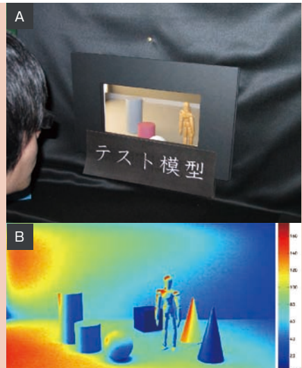
【左写真】 A) 模型空間を用いた照明の心理評価実験 B) 輝度の空間分布の定量的な分析 【右写真】 ステージにおける三次元的な音響性状を計測し、三次元音場再現システムを用いて評価する
