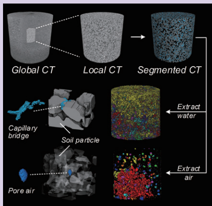
【左図】排水過程における土中間隙流体の形態変化の可視化
