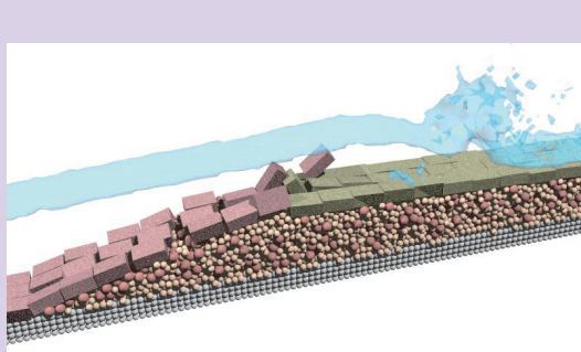
【左図】高波による潜堤の被災シミュレーション 海岸景観に配慮した水没型の防波堤である潜堤は、捨石を積み上げたマウンドとコンクリートブロックから構成される。左図は、高波が砕波して生じる流れによる潜堤の崩壊過程を再現した数値シミュレーションの結果である。
