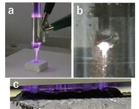
放電技術を使ったナノカーボンの高機能化装置 3 選： (a) プラズマトーチによってグラフェンに細孔を空け分子フィルターをつくることが出来ます。 (b) 水中アーク放電によってグラファイトからカーボンナノホーンを合成することが出来ます。 (c) カーボンナノチューブ膜に大気圧バリア放電処理を行って表面の活性化を行い、高性能の電池電極をつくることが出来ます。
