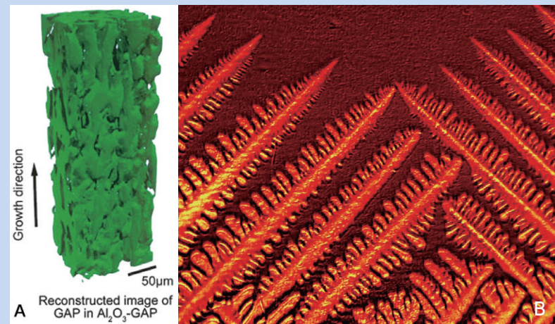
シンクロトロン放射光を利用した 3 次元組織形態の直接観察
