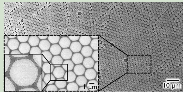
大小 2 種類の微粒子から構成される規則配列単層膜 規則的な粒子配列構造は特異な光学的性質を示すため、簡単に、かつ大面積に粒子膜を作製する方法とそのメカニズムを研究しています。この写真では、小粒子（直径 45 nm）が大粒子（直径 2 μm）同士の隙間に入り込むことで、大粒子が規則的に配列するのを助けています。
