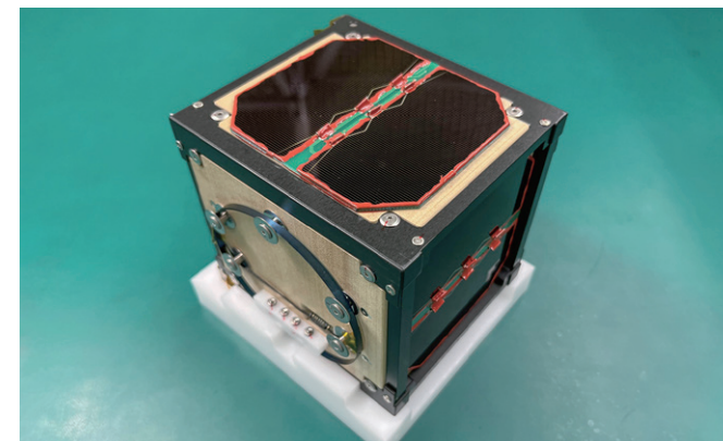
世界初の木造人工衛星「LignoSat」
