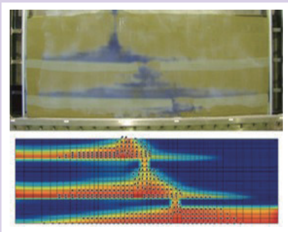
【左図】排水過程における土中間隙流体の形態変化の可視化
