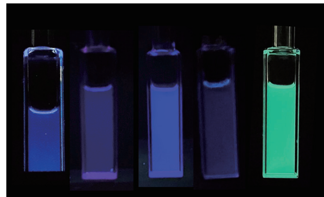
分子の特定の位置の置換基を変えるだけで発光色が変化している様子
