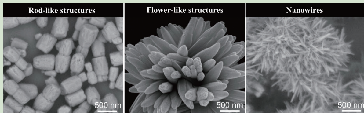
様々な形状の ZnO ナノ結晶
