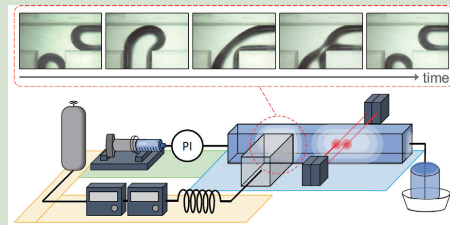
マイクロデバイスにおける二相スラグ流生成制御・モニタリング マイクロデバイスは新しい生産装置として注目されています。“control by design”の考え方に基づくスラグサイズ制御法、圧力データ解析による運転状態監視法を開発しています。
