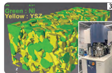
1. 太陽光水素製造のための高効率光触媒および光電極の開発 2. 酸化物(セラミックス)にはない革新的な機能を示す複合アニオン化合物 3. 集束イオンビーム走査電顕(右図)と電極の三次元再構築画像
