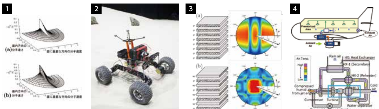
1 ボルツマン方程式に基づいて解析した物体面上における摂動速度分布関数の特徴 (a) 凸面の場合, (b) 凹面の場合 2 未知環境下での探査ローバーの制御実験 3 航空宇宙機の構造に用いられる繊維強化複合材料の異方性弾性特性 (超音波による測定結果) (a) 一方向積層材, (b) 直交積層材 4 航空機用空調システム
