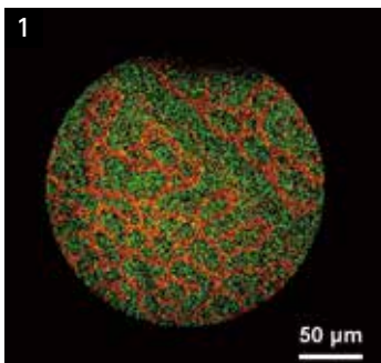
1 透過型二次イオン質量分析による有機物試料の分子イメージング
