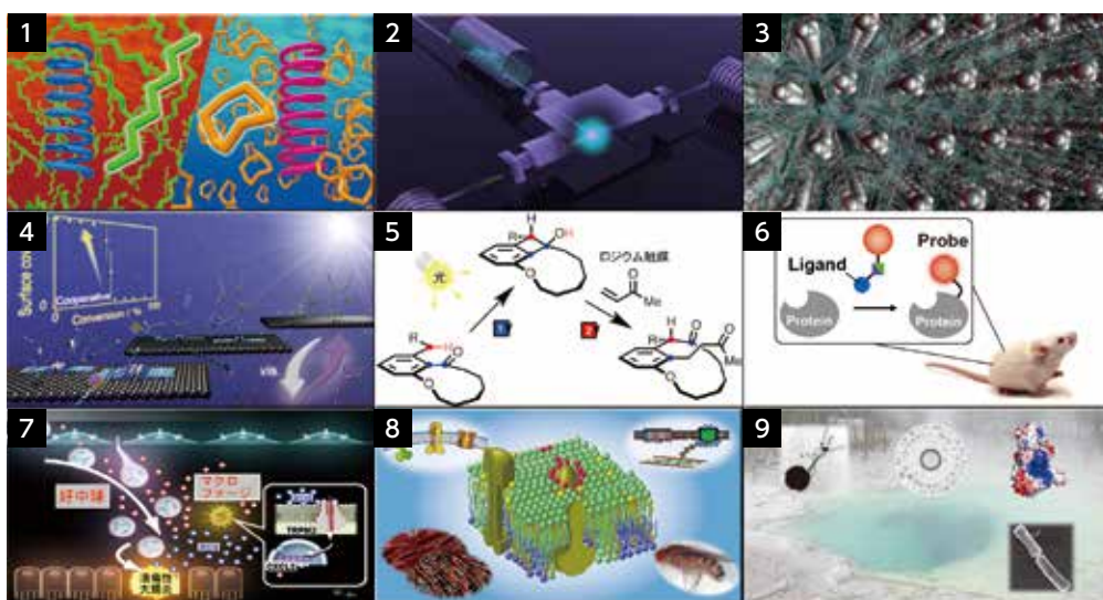
1 溶媒効果のわずかな違いを増幅するらせん高分子 2 フラスコではできない化学合成を可能にするフローマイクロリアクター 3 柱型環状分子ピラー [n] アレーンからなる分子空間材料 4 二次元界面における分子配列の光コントロール 5 オルトシクロファンからメタシクロファンへの環拡大 6 アフィニティー駆動型反応による選択的なタンパク質化学修飾 7 炎症性細胞を呼びよせる \text{Ca}^{2+} 流入チャネル TRPM2 8 生命現象を統御する脂質分子群 9 極限環境微生物のゲノム微生物学
