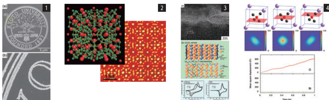
1 走査プローブリソグラフィによる有機単分子膜の選択的分解、フッ酸によるエッチング、及び無電解めっきを経て形成された金 (Au) によるクスノキマークパターン 2 熱電変換クラスレート化合物の結晶構造モデルと、高分解能走査透過型電子顕微鏡 (STEM) 像 3 (a) LiCoO 2 正極-La 2/3-x Li 3x TiO 3 (LLT) 固体電解質からなる全固体リチウム二次電池モデルセルの正極/電解質界面の高分解能透過電子顕微鏡像、(b) LiCoO 2 正極-La 2/3-x Li 3x TiO 3 (LLT) 固体電解質間の結晶方位関係、(c) モデルセルの電気化学特性。界面におけるアモルファスLLT領域の形成により充放電サイクル安定性が向上 4 第一原理分子動力学法を用いた立方晶Bi 2 O 3 の酸化物イオン伝導度シミュレーション
