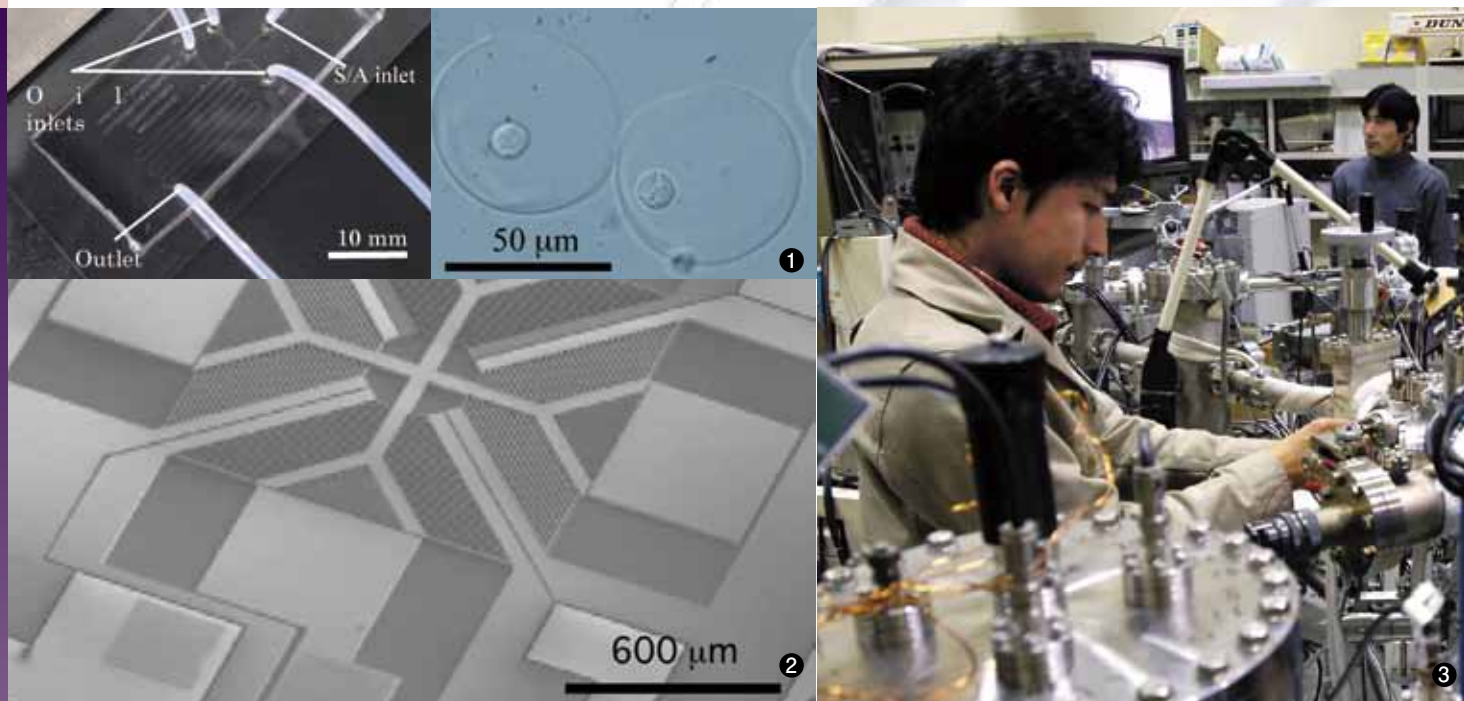
①細胞カプセルングルビーズのためのマイクロ流路デバイスおよび作製されたゲルビーズ（細胞を内包している）
