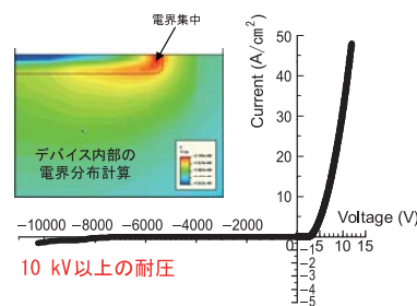
10 kVの耐圧を有するSiC pnダイオードの実現
