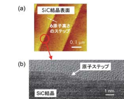
(a) SiC半導体結晶表面の原子間力顕微鏡像 (b) SiC結晶断面の透過電子顕微鏡像 共に、表面に6原子高さの原子ステップが形成されていることが分かる。
