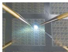
InGaN窒化物半導体マイクロファセット量子井戸構造を利用した多波長LED
