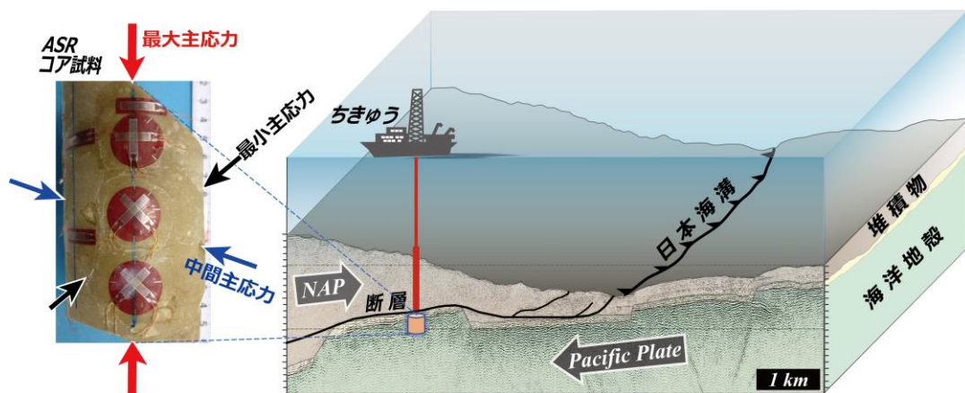
図 1 東北地方太平洋沖地震後の震源断層直下の応力状態。応力計測用の ASR コア試料(左)は海底下深度約 828 m(プレート境界断層の深度より約 8 m 深)から採取されたもので、円柱表面に貼ってある赤茶色のものはひずみ測定用のセンサーである。図中の NAP は北米プレート(North American Plate)の略である。
